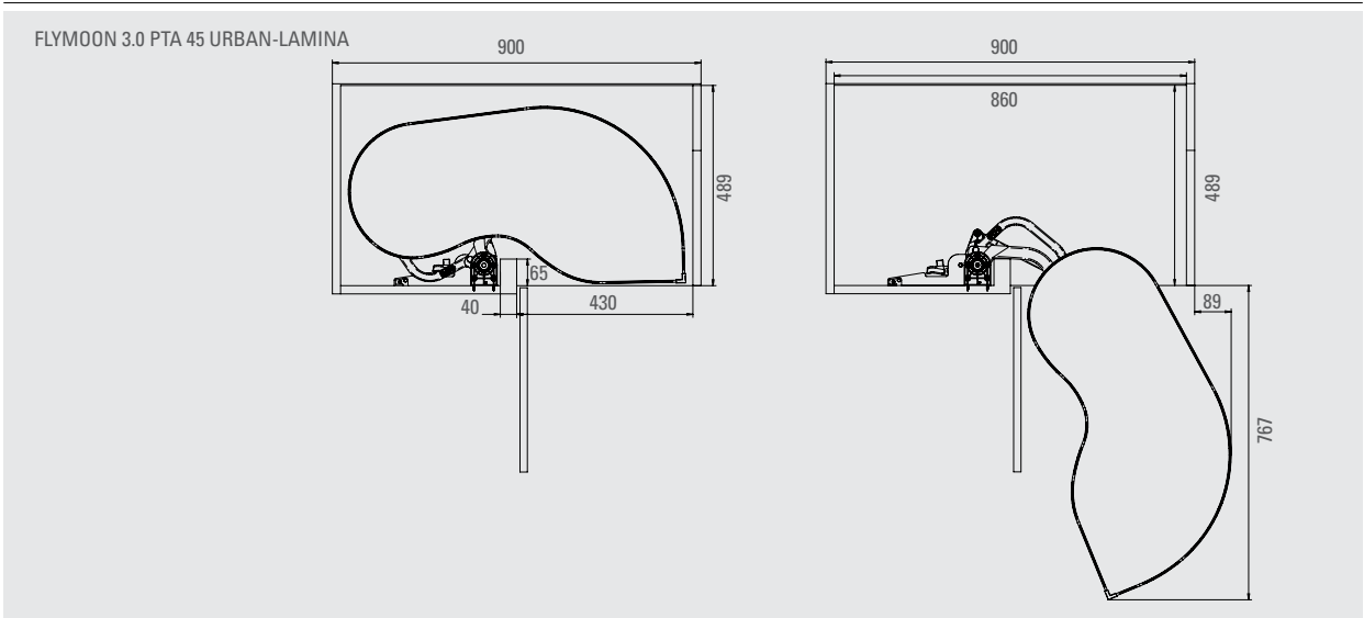
HOJA DE MONTAJE SET 2 PIEZAS MONTAJE
