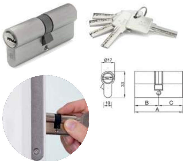
Cilindro de seguridad 6 pins+5 llaves de seguridad latón
