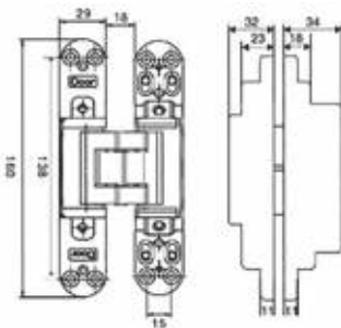
Bisagras ocultas de 3 regulaciones Incluye tornillos inox. para el montaje. La bisagra no tiene mano, independientemente para izquierda y derecha Invisible hinge with 3 regulations Including stainless steel screws for mounting. Regardless of left and right hinge
