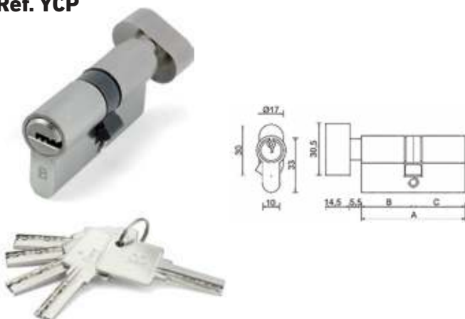
Cilindro de seguridad con pomo 6 pins+5 llaves de seguridad latón
