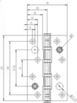
Bisagra de seguridad canto cuadrado, remate corto con 4 rodamientos Security hinge with square edge, flat tip, 4 ball bearings
